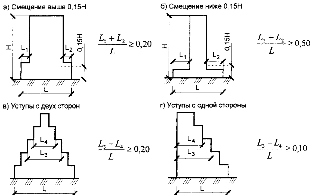
Рисунок 1. Признаки не регулярных зданий
